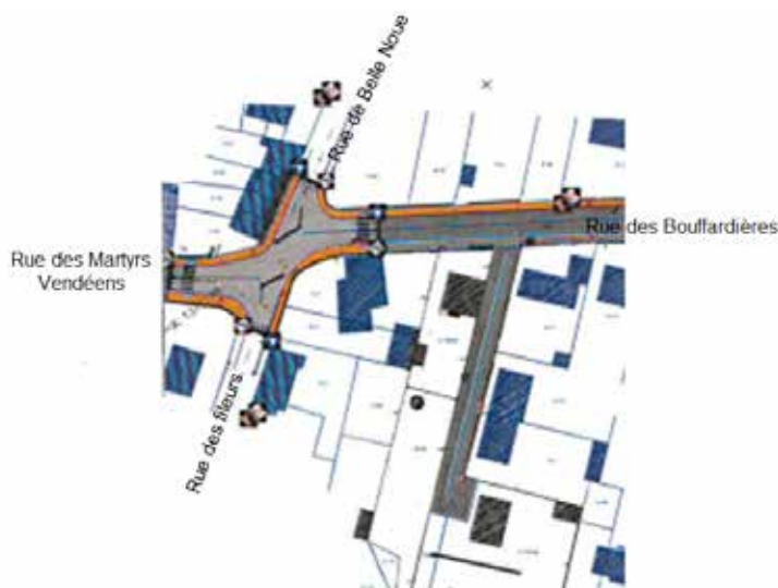
Plateau de surélévation au niveau du carrefour
